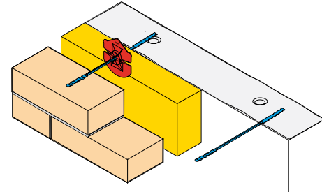
2. Lijm-lijmspouwanker
