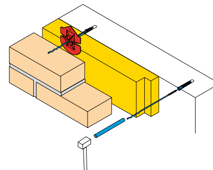
9. Kopgevelanker
