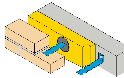
3. Prefab-lijmspouwanker
