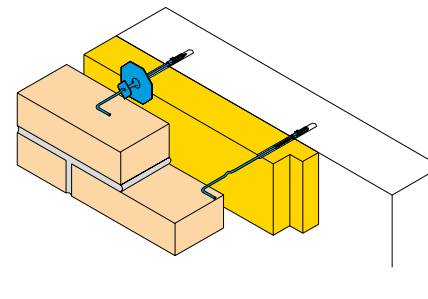
9. Kopgevelanker
